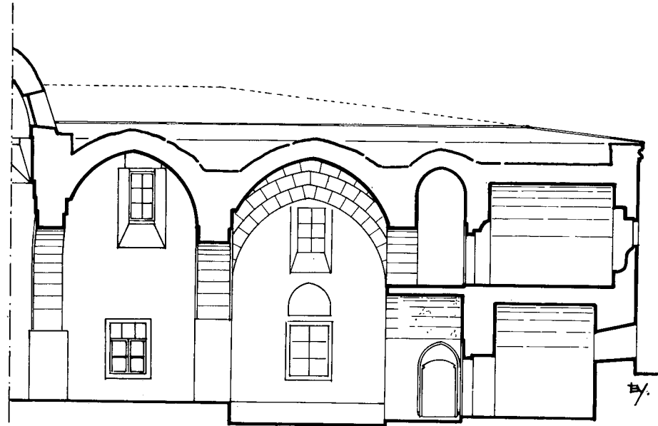
Çizim : 11 C - C Kesiti
