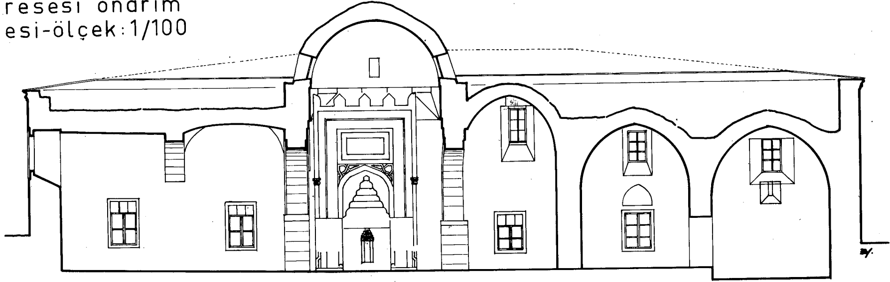
Çizim : 9 A - A Kesiti
