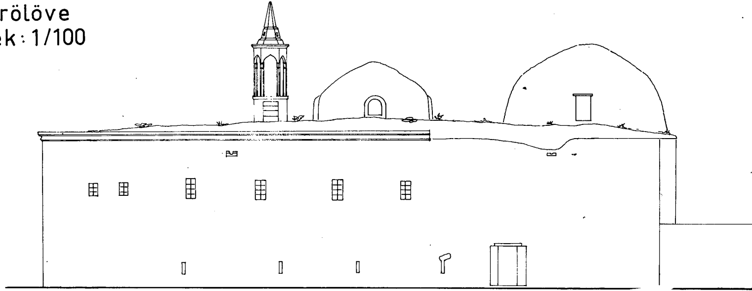
Çizim : 6 Batı cephesi
