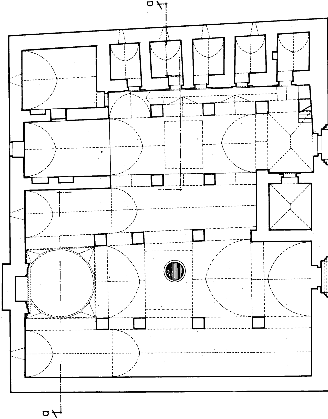
Çizim : 17/a Cami ve medrese alt kat plânı
