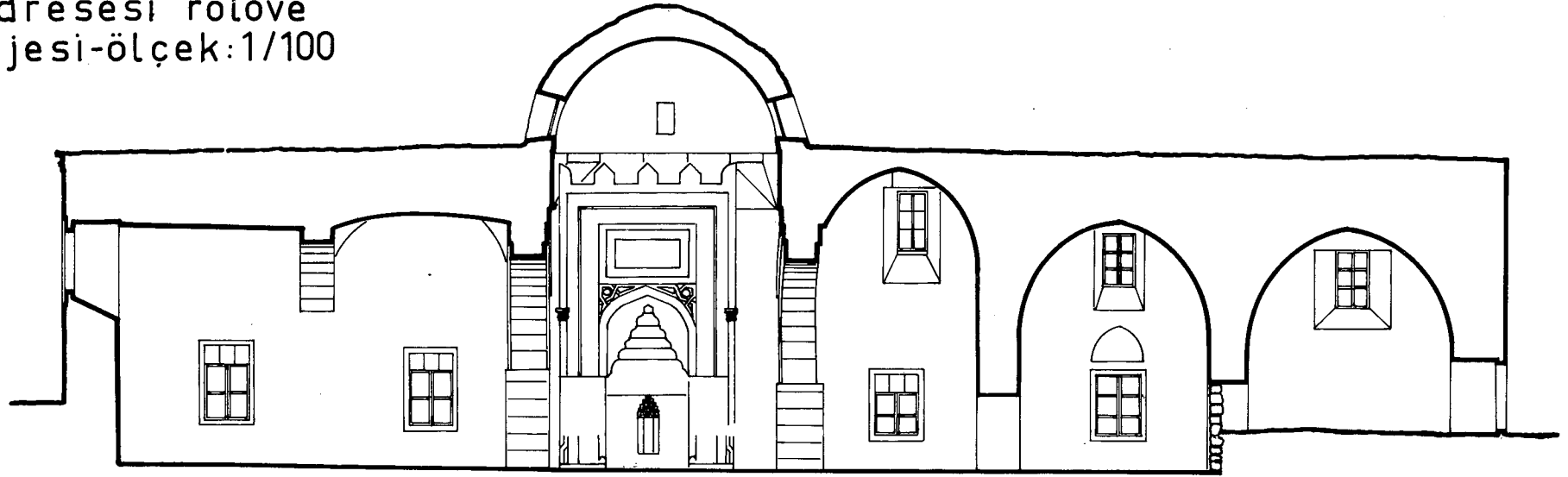
Çizim : 2 A - A Kesiti
