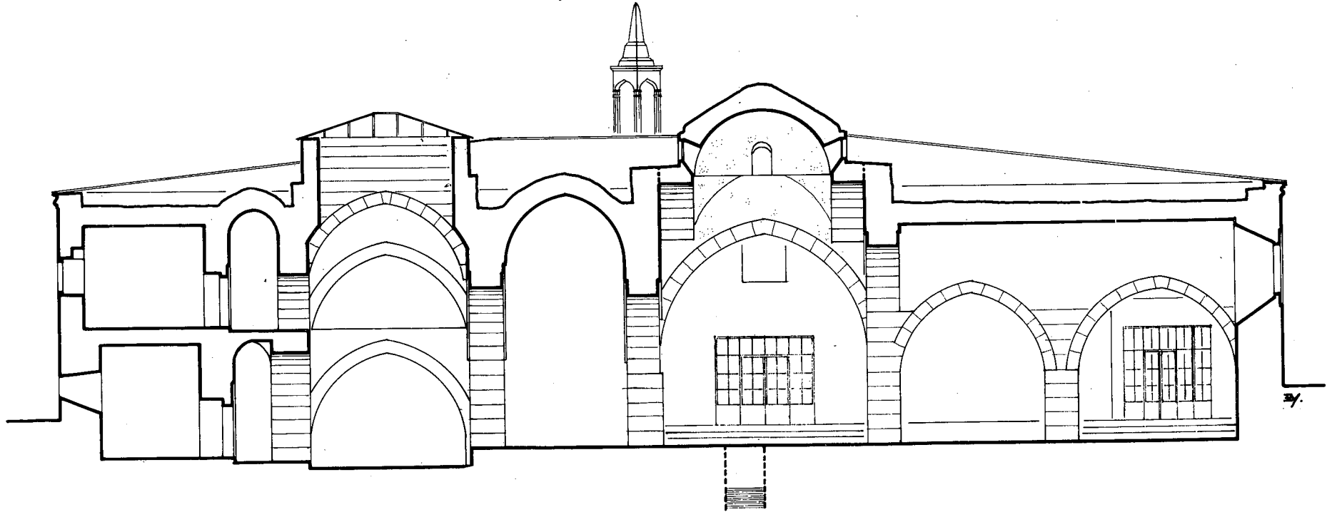
Çizim : 10 B - B Kesiti
