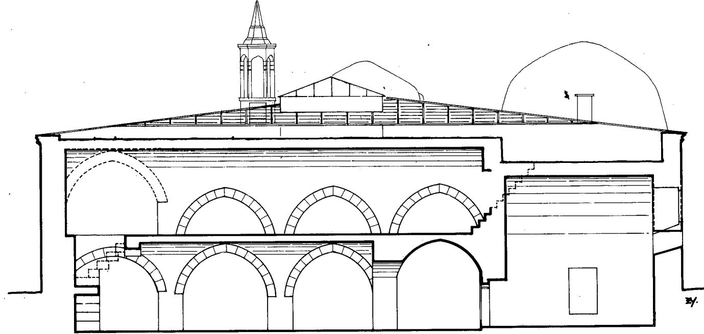
Çizim : 13 E - E Kesiti
