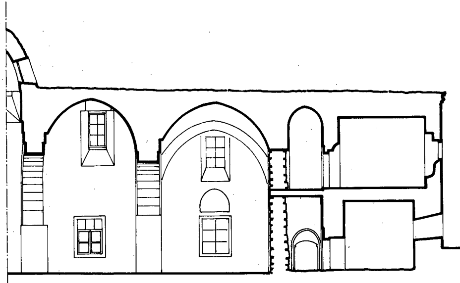
Çizim : 4 C - C Kesiti
