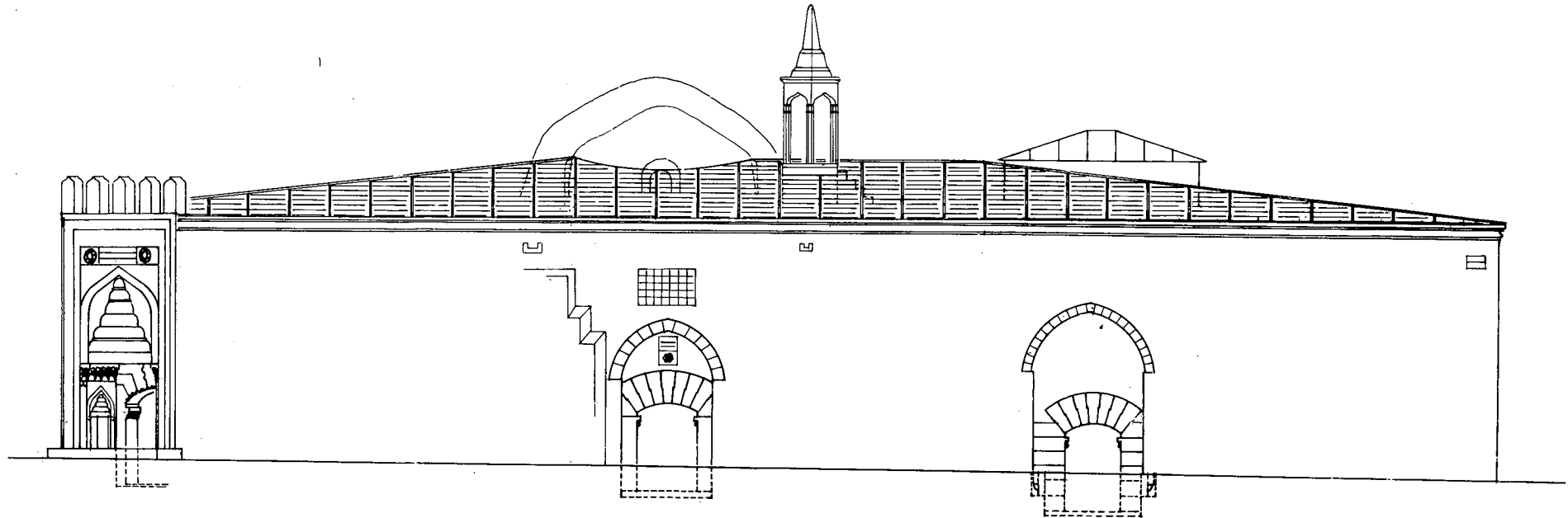
Çizim : 16 Kuzey cephe
