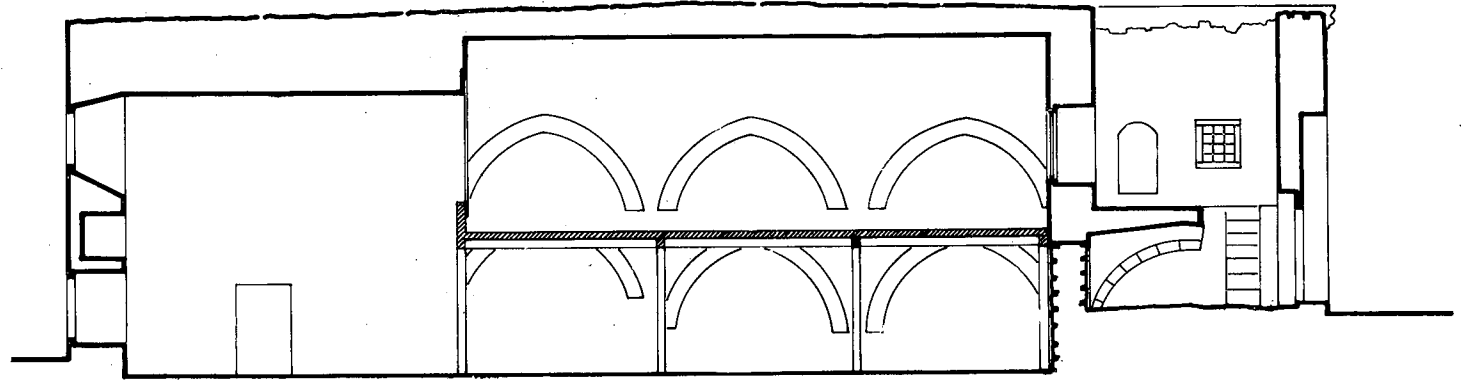
Çizim : 5 D - D Kesiti
