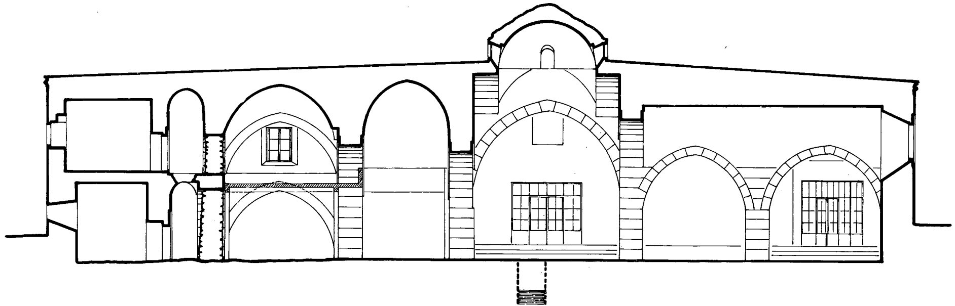
Çizim : 3 B - B Kesiti
