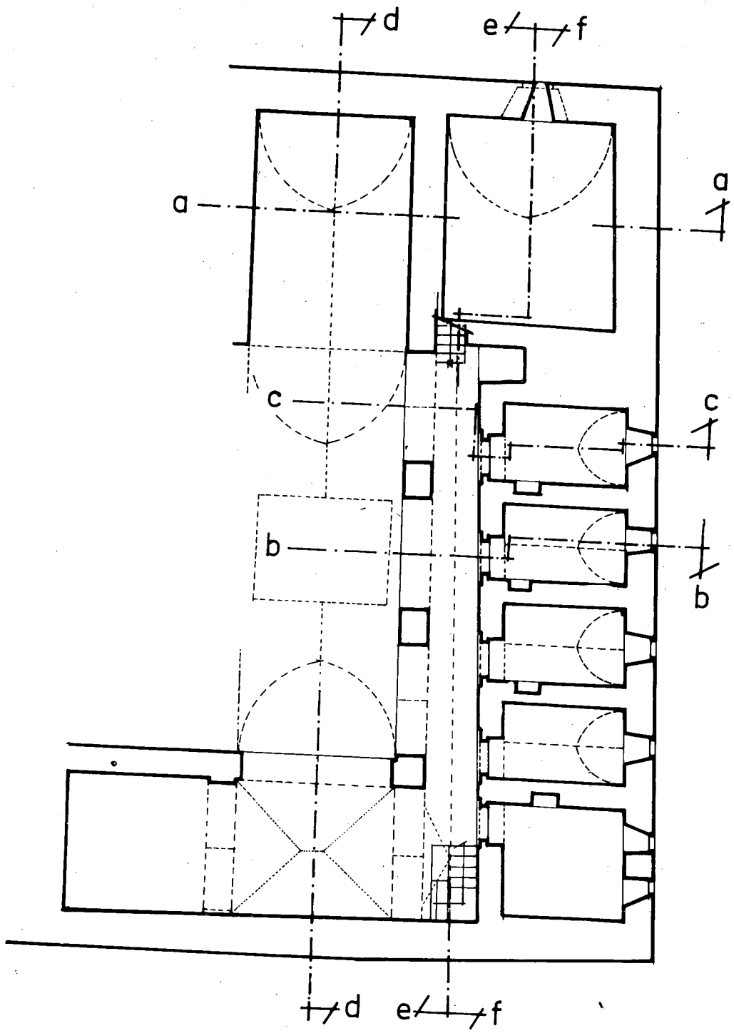
Cizim : 8/b Medrese üst kat plânı
