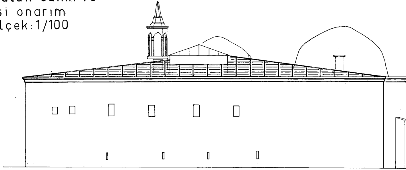
Çizim : 15 Batı cephe
