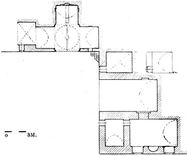
Plân : 2. Marufiye Medresesi.
