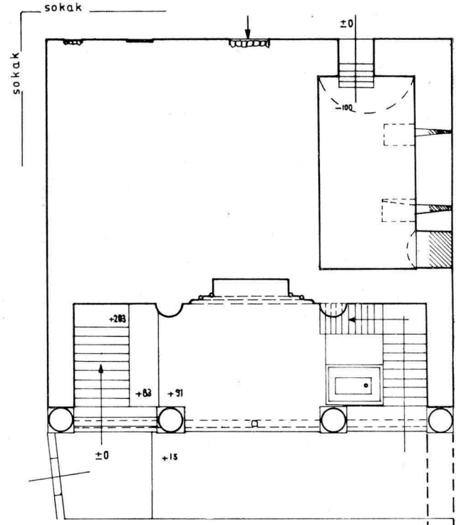
KONYA BULGUR TEKKESİ MESCİDİ zemin planı / aralık 1970 ara altun
