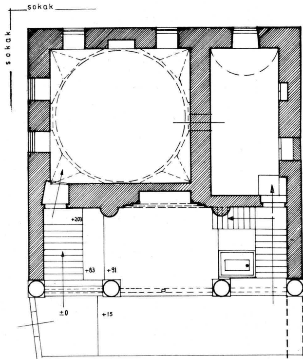
KONYA BULGUR TEKKESİ MESCİDİ mescit katı planı / aralık 1970 ara altun
