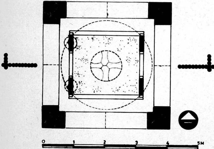
Şekil 3 Erzurum'da Mahmud Paşa Türbesi Planı
