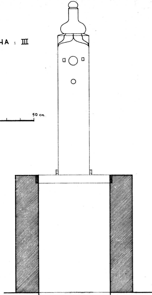
Takkeci İbrahim Ağa Sebilindeki kuyu bileziğinin rölövesi.
