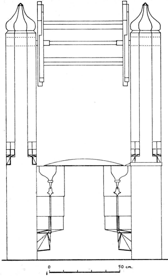
Bayram Paşa külliyesindeki kuyu bileziğinin rölövesi.
