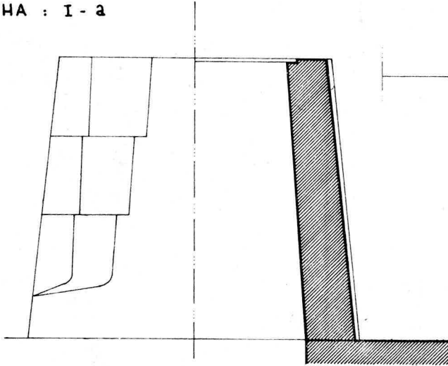
Zal Mahmut Paşa Medresesindeki kuyu bileziğinin rölövesi.
