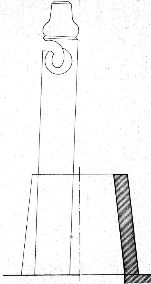
Yedikule'de Kule Meydanı sokađı bařındaki kuyu bileziđinin rölövesi
