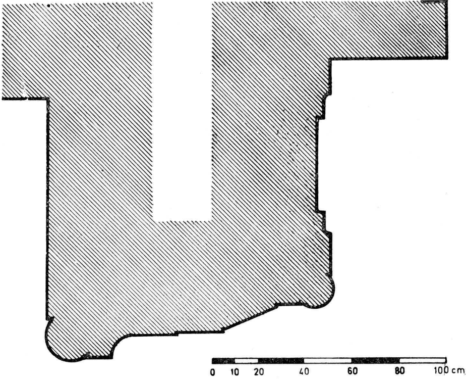
Şek. 4- Taçkapı profili Fig. 4- Le profil du portail
