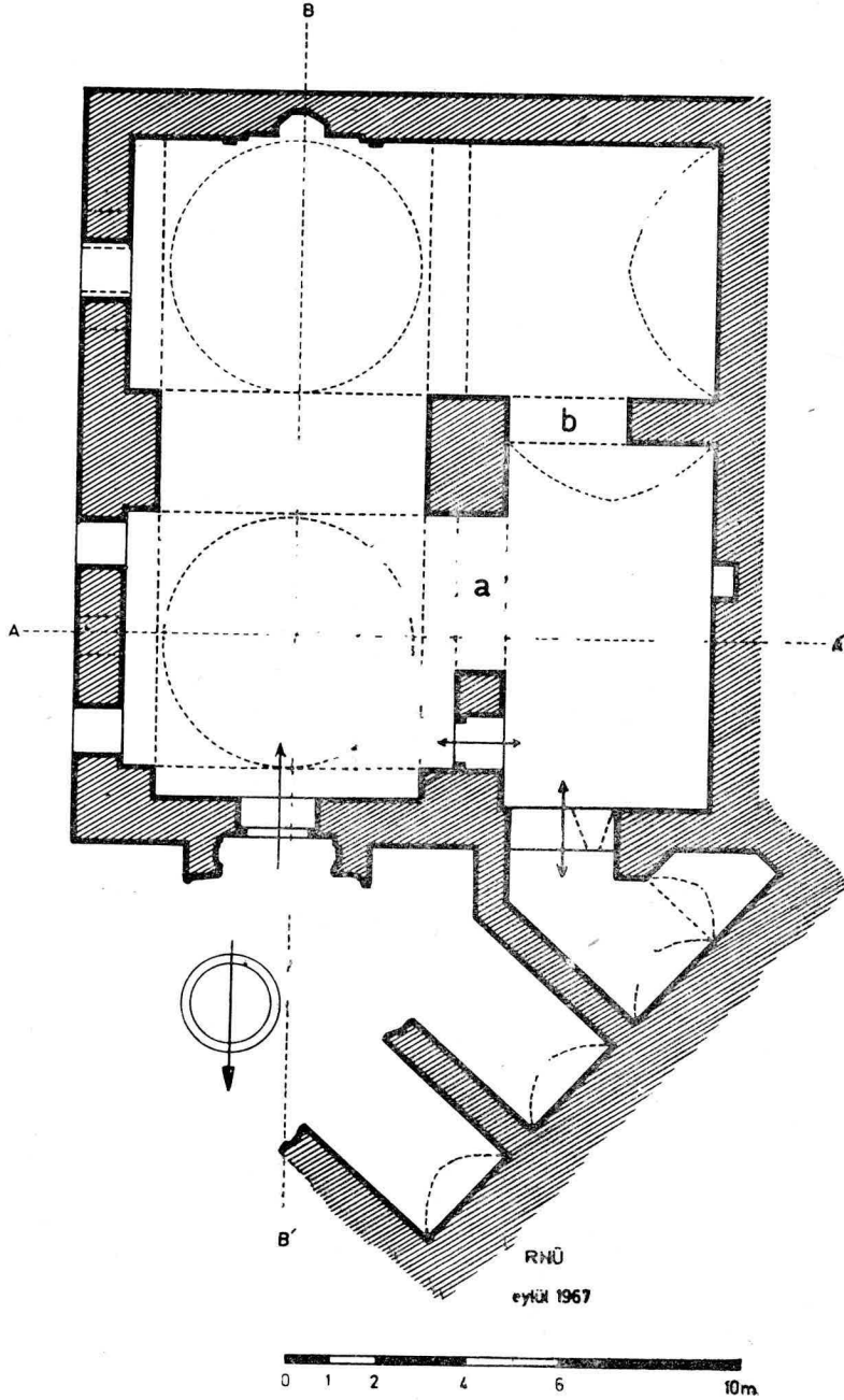
Şek. 1- Zaviyeli Cami. Plan
