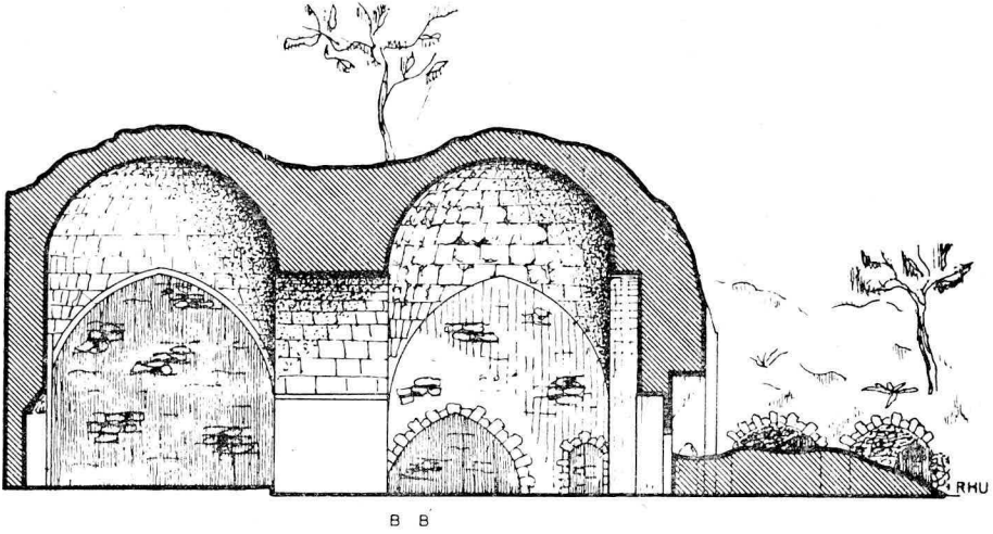
Şek. 3- B-B' kesiti
