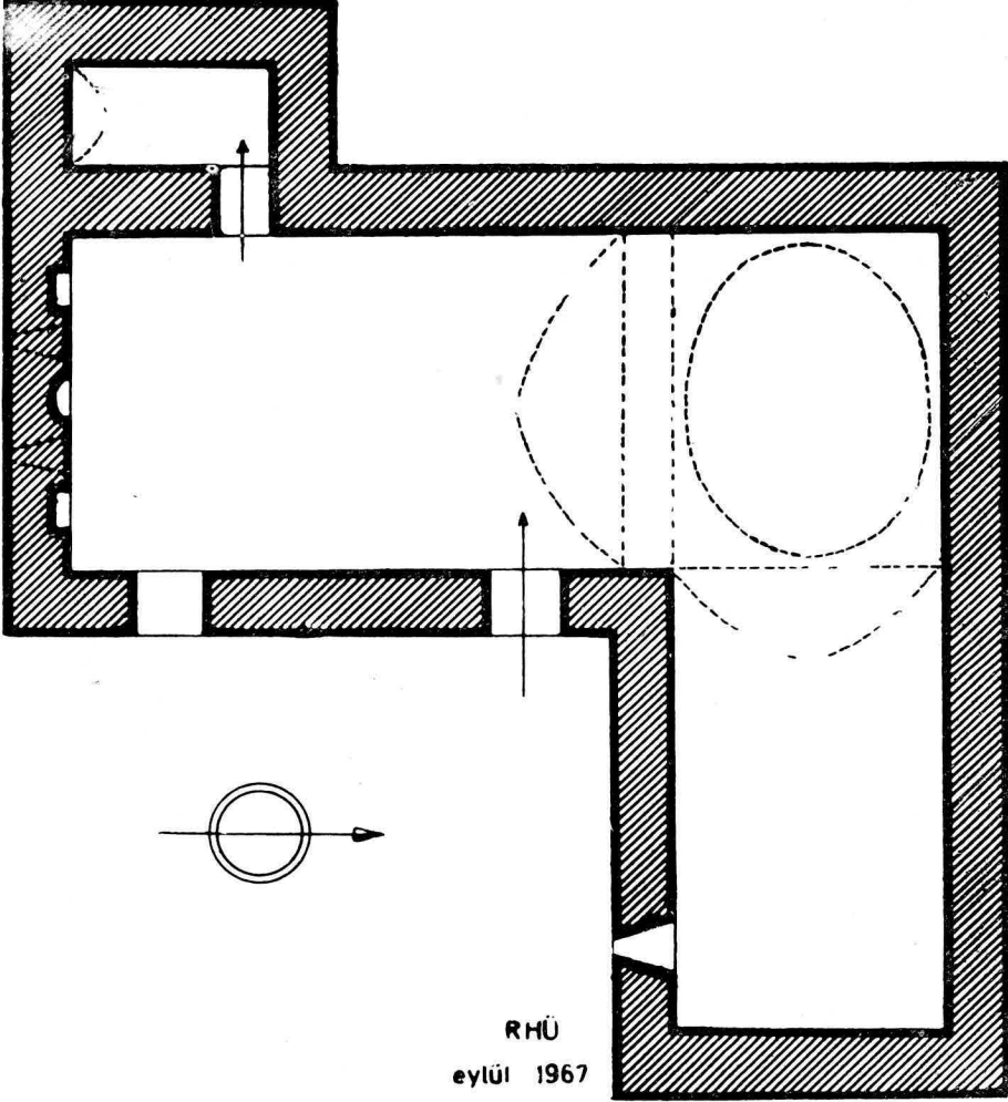
Şek. 12- Hankâh. Kroki Fig. 12- Le Croquis du Hanqah.
