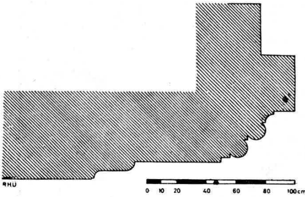
Şekil 2. Kervansaray, Taçkapı profili.
