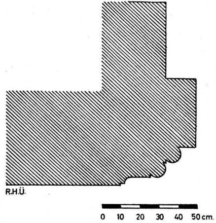
Şekil 3. Kervansaray, İçkapı profili.
