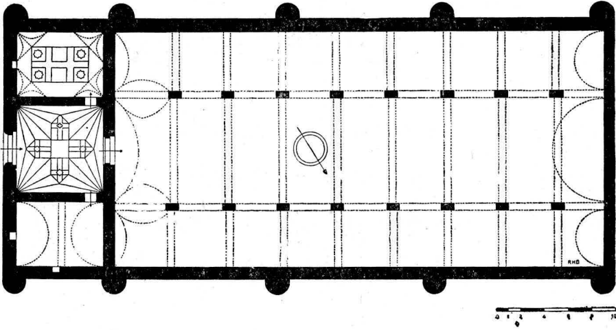
Şekil 1. Iğdır Kervansarayı, plân.
