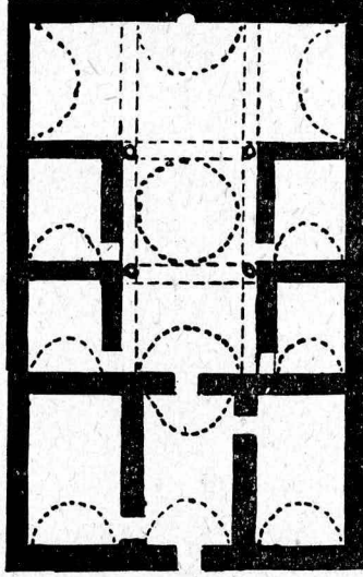
Şekil: 18 — Afyon — Şincanlı — Boyalıköy : medresenin plâni.
