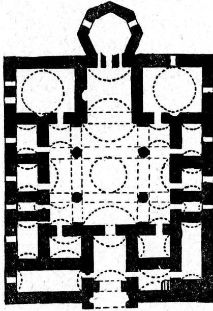
Şekil : 9 — İsparta — Atabey : Ertokuş Medresesi plânı.
