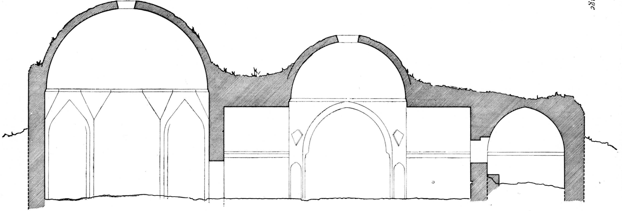
A-A KESİTİ
