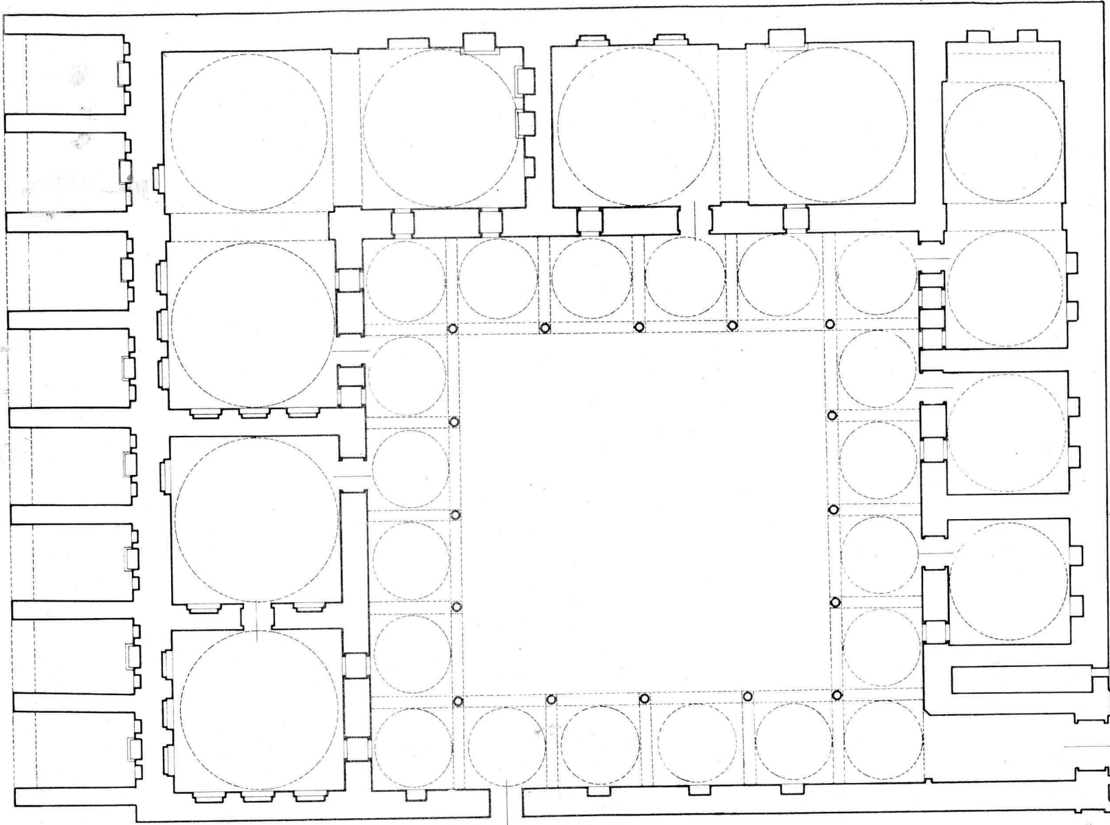
Manisa — Muradiye Külliyesi İmareti Plân Projesi
