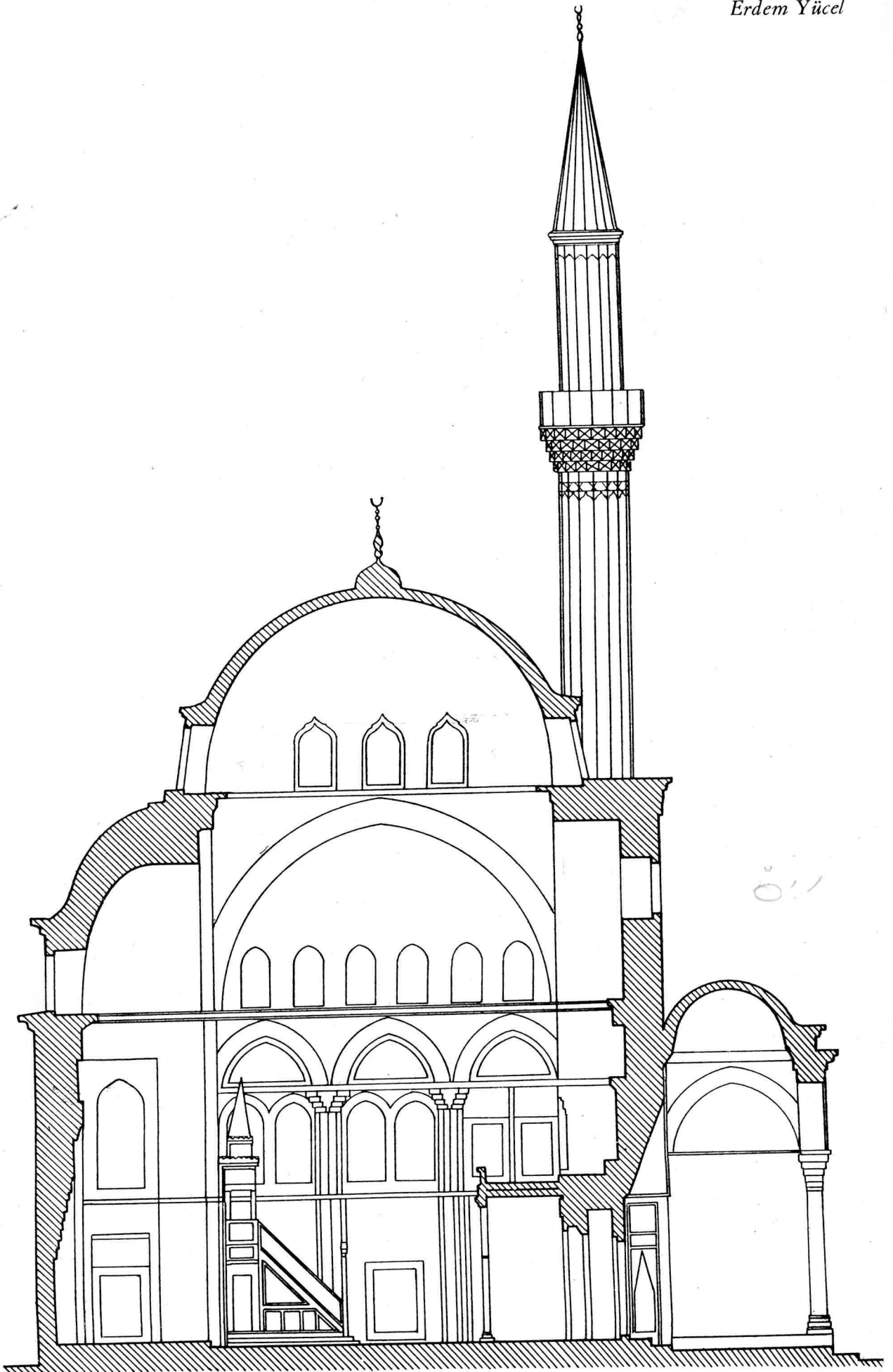
Manisa — Muradiye Camii A-A Kesiti.
