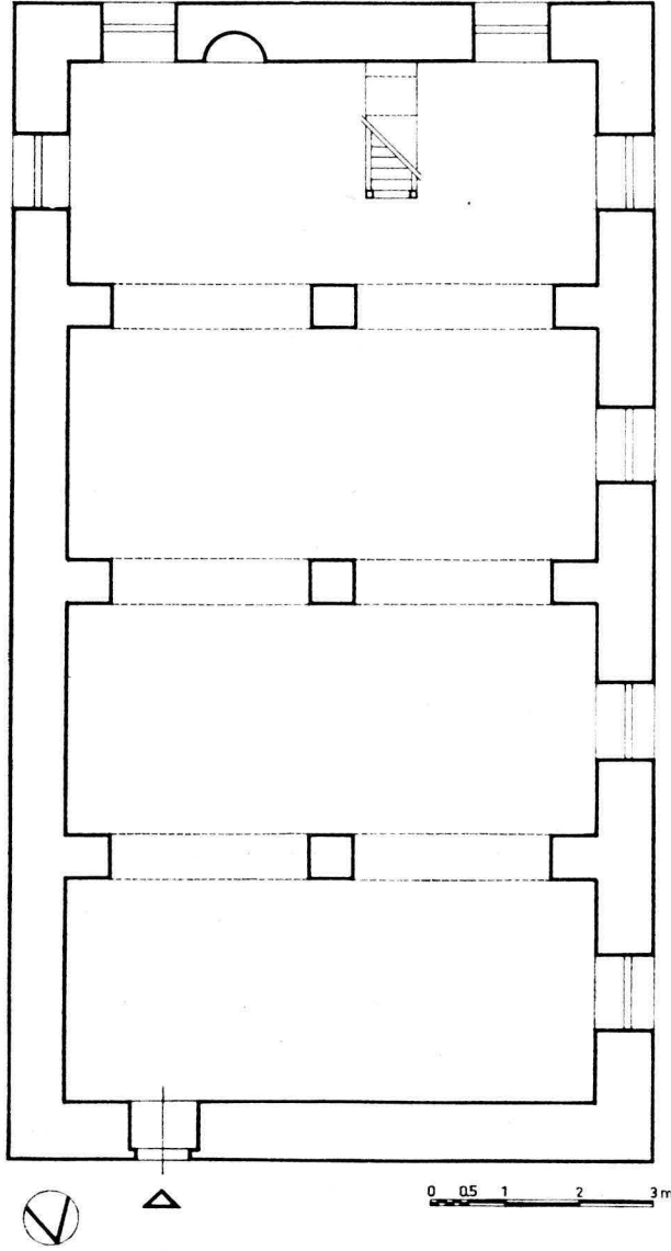
Şekil 2. Ulukale Yusuf Paşa Camisi'nin planı.
