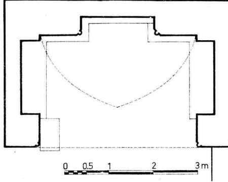
Şekil 5. Ulukale Köy Meydanı Çeşmesi'nin planı.
