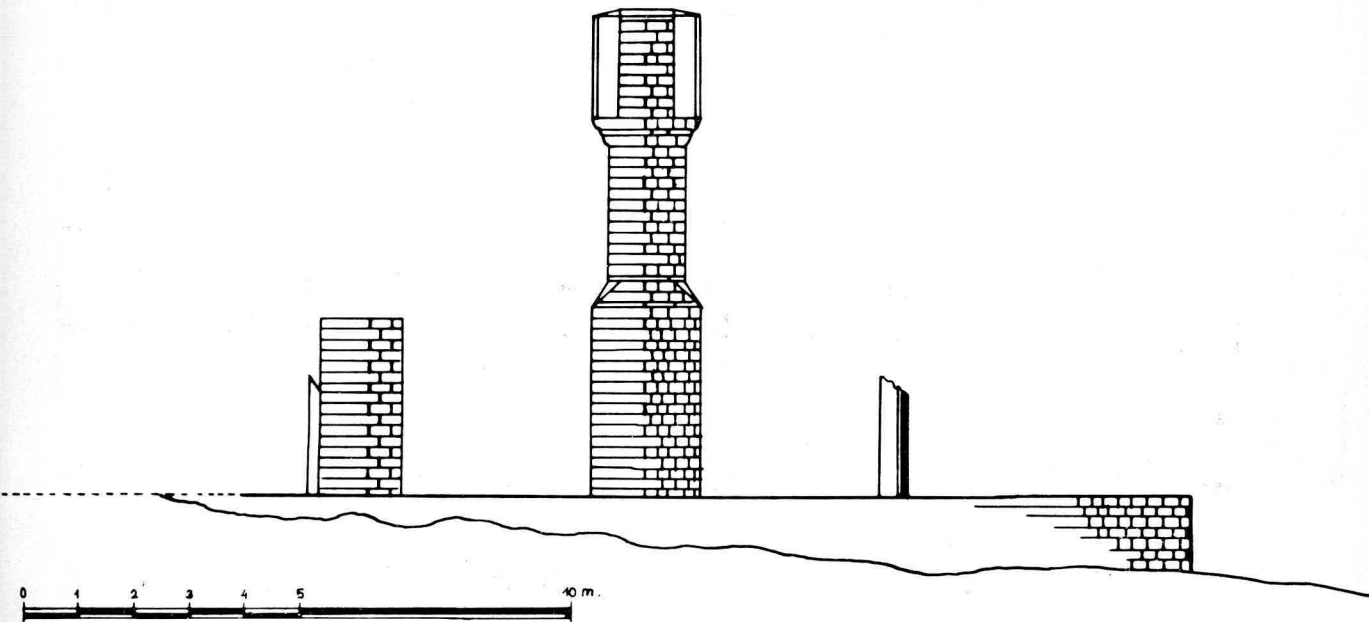
Çizim : 3/a — Haznedarlı Camisi, uzunlamasına kesit
