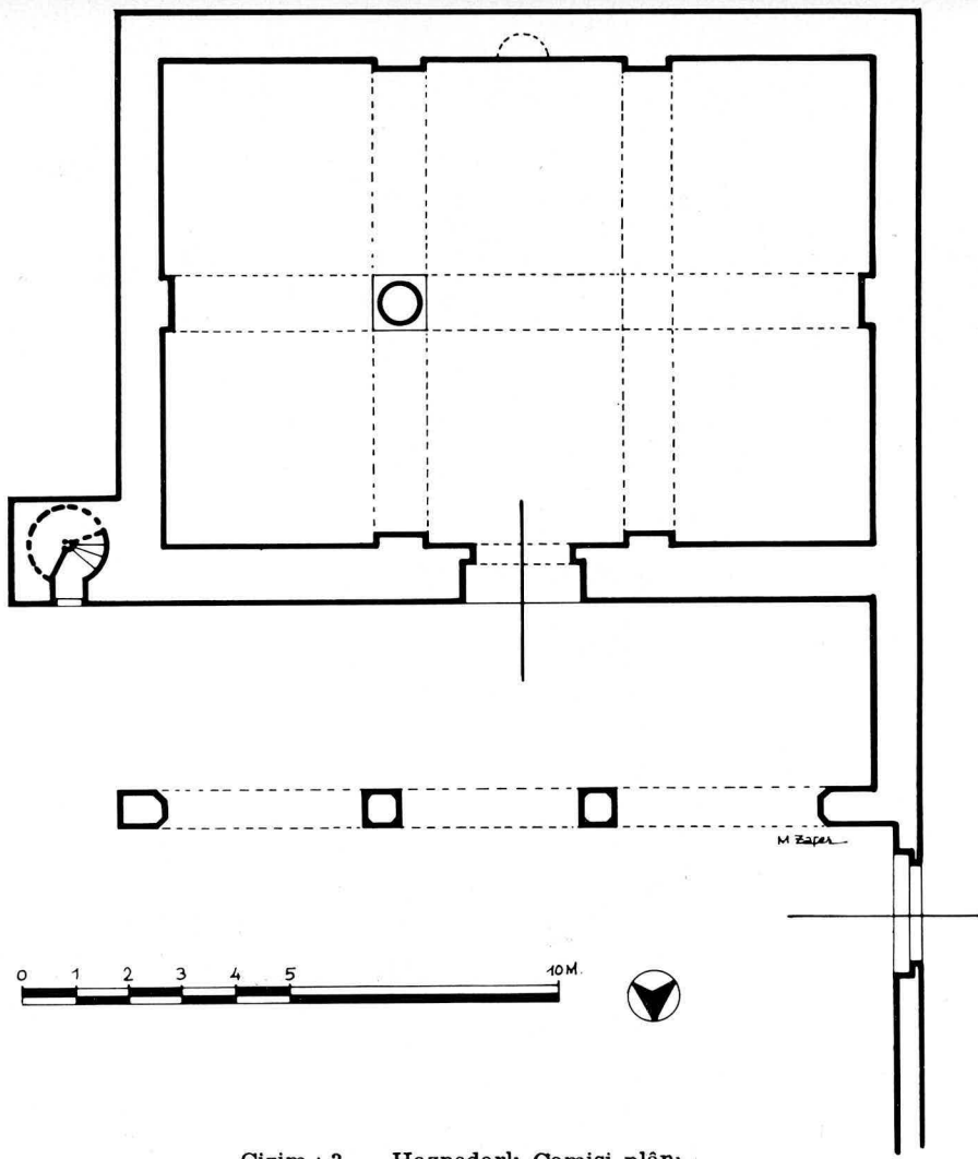
Çizim : 3 — Haznedarlı Camisi plânı
