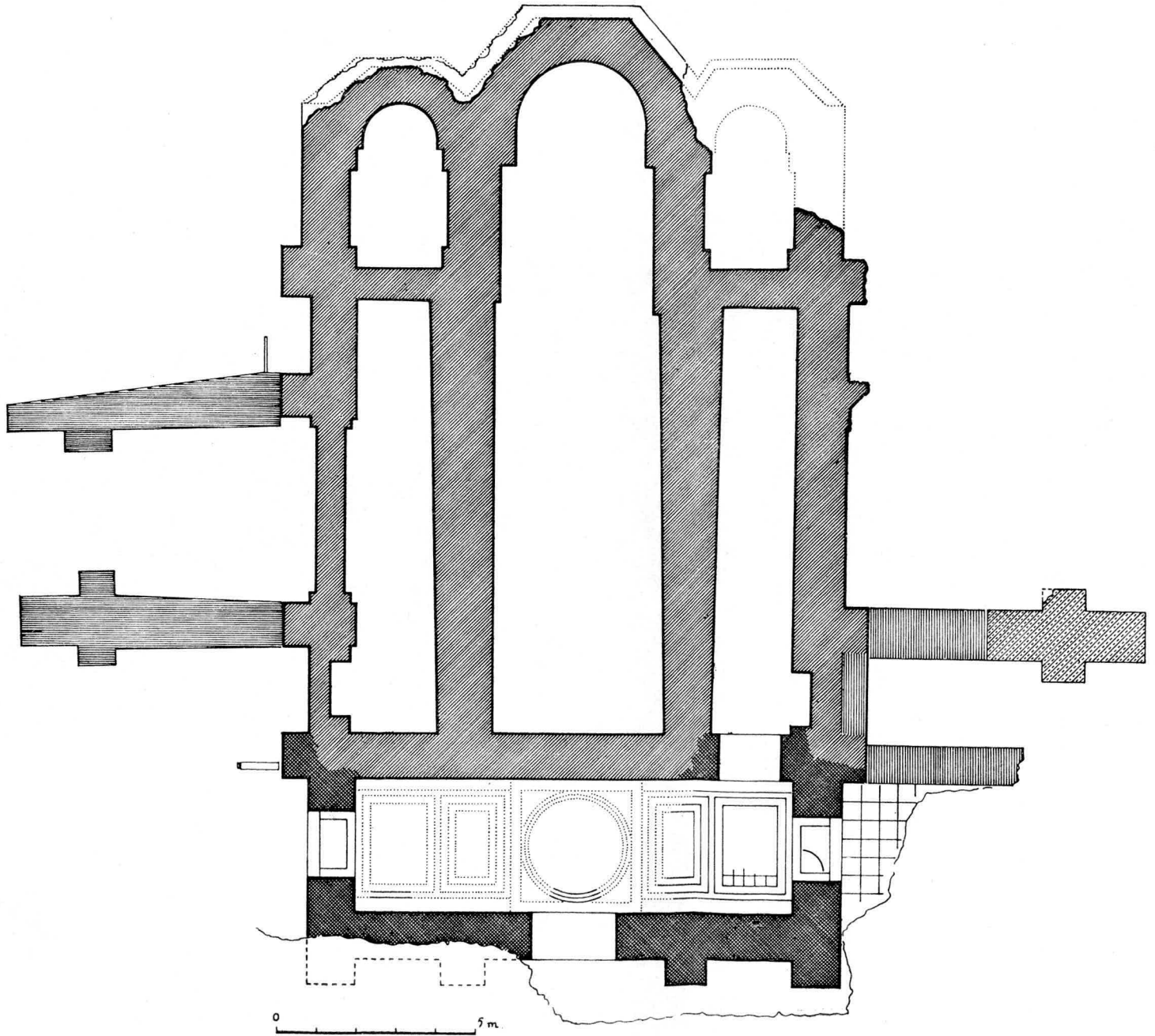
Resim 47. Kalıntı'nın buluntu rölövesi (Çizen : Y. Önge).
