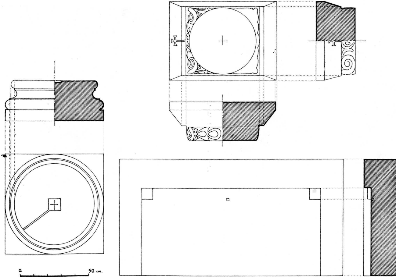
Resim 36. Sütun başlığı, kaidesi ve eşik deseni (Çizen : Y. Önge).
