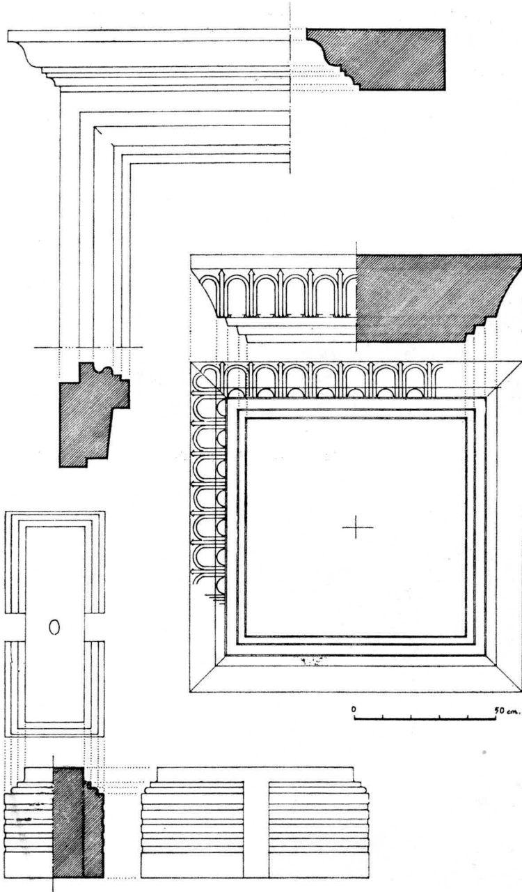
Resim 31. Paye kaidesi, kapı çerçevesi ve entablement'ların deseni ve kesitleri (Çizen : Y. Önge)
