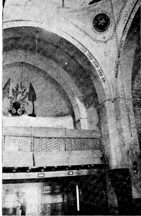
Resim 20 - 21 - Kubbe ve örtü sistemi detayları
