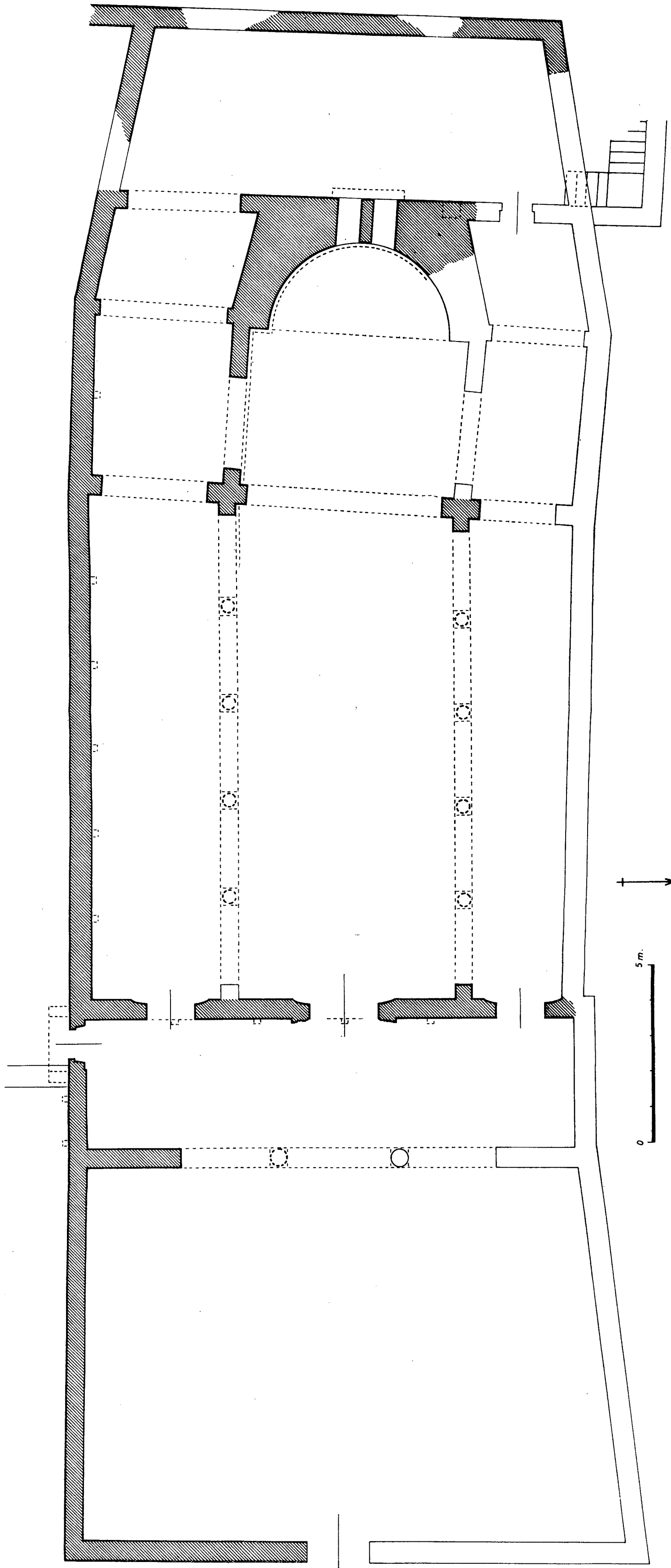
Res. 27 — IV. No.lu basilikanın yeni plânı (çizen : Yılmaz Önge).
