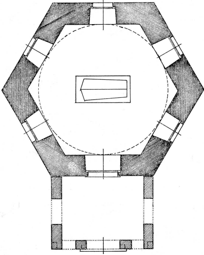
PLAN_ ö. 1/100
