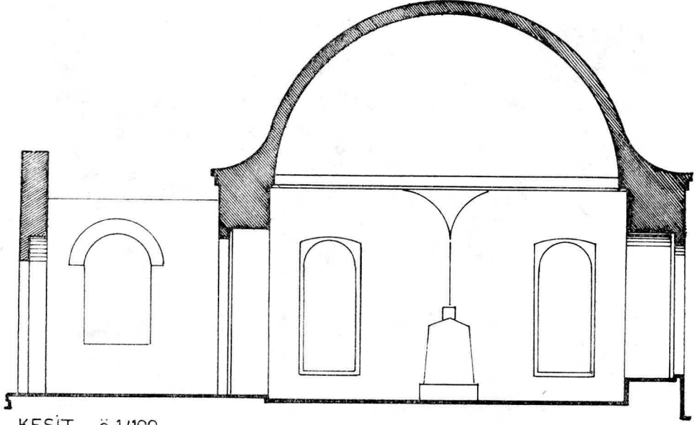
KESİT _ ö.1/100
