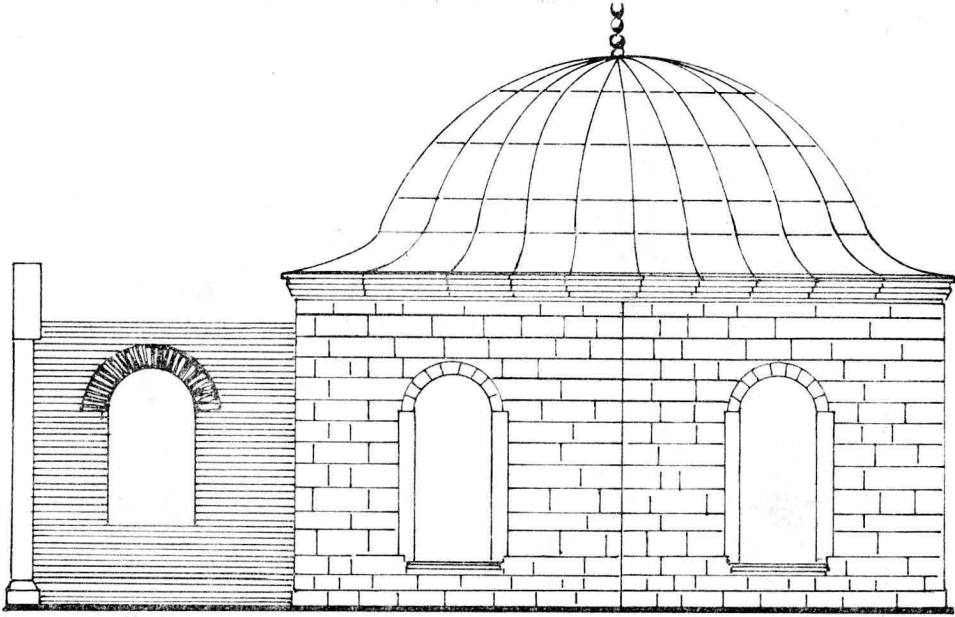
YAN GÖRÜNÜŞ _ ö.1/100
