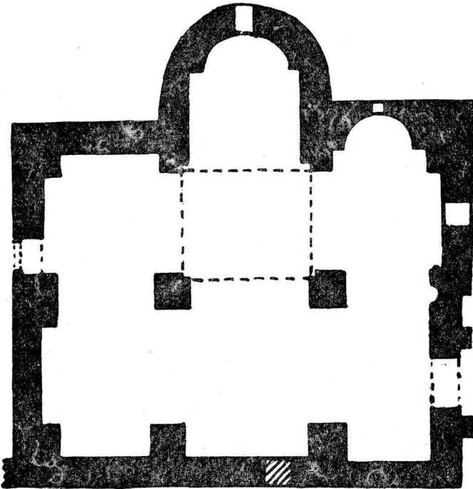
Res. 22 — Eflâton mescidi olan kilisenin plânı (Ramsay ve Bell'in kitabından).
