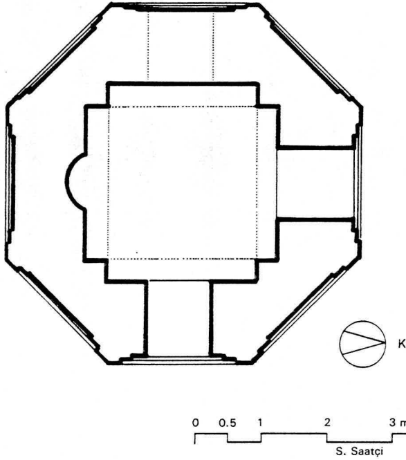
Şekil 1 — Türbenin planı.
