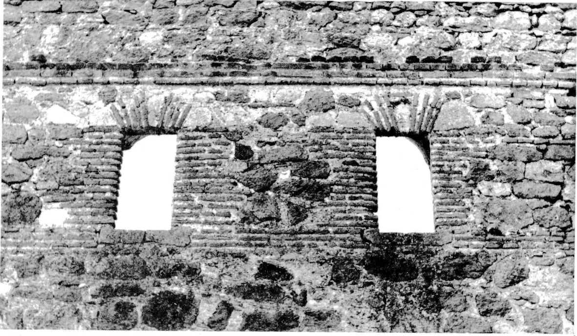
RESİM: 12 Doğu cephesinde, cephe dokusu ve fuğla kornisi gösteren detay.
