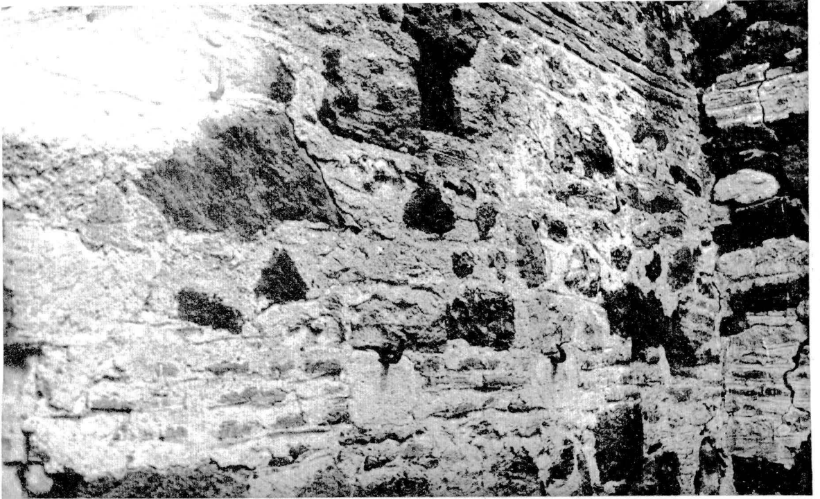
RESİM: 10 Beden duvarlarına yerleştirilmiş taşıyıcı askı demirleri.
