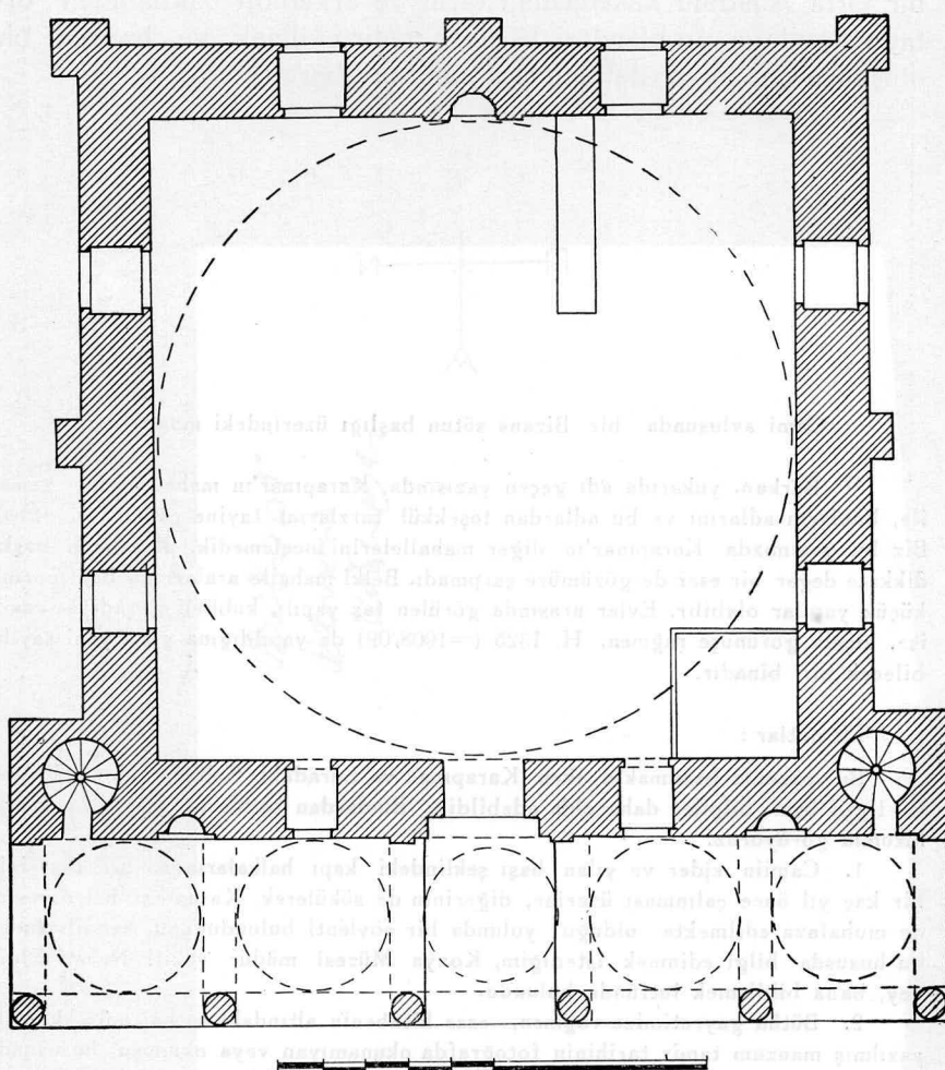
Sultan Selim camii'nin plânı
