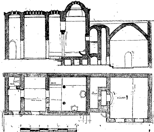
Hamamın plânı ve kesimi
