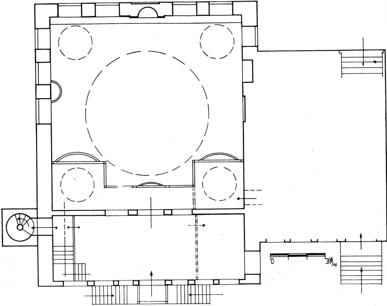
İSTANBUL/KULELİ , KULELİ OCAĞI (Mahmut Han) MESCİDİ plan krokisi kasım 1970 a.altun
